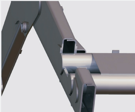
Nueva concepción de los perfiles "U"
